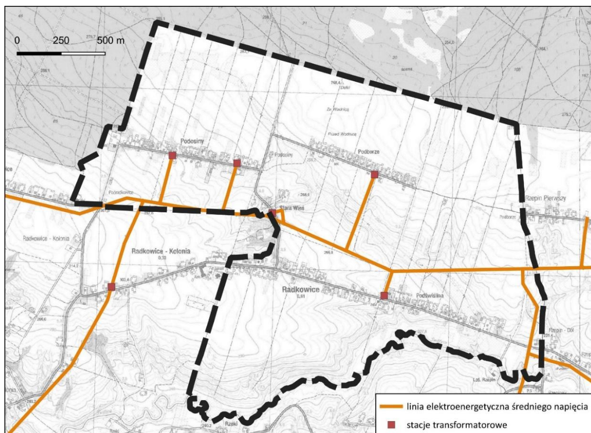
Rysunek 10. Przebieg linii elektroenergetycznych na terenie opracowania
